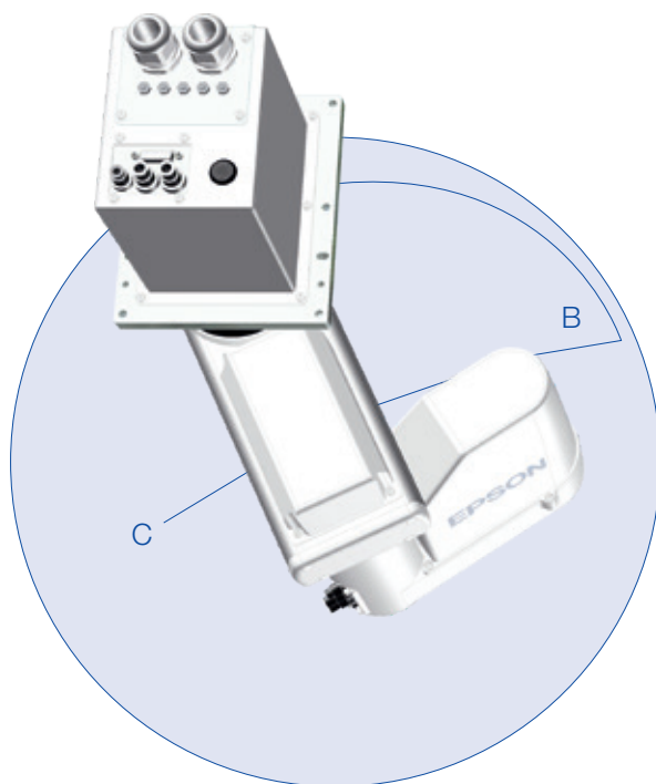
Epson Spider Roboter: Zylindrischer Arbeitsbereich ohne Totzone
