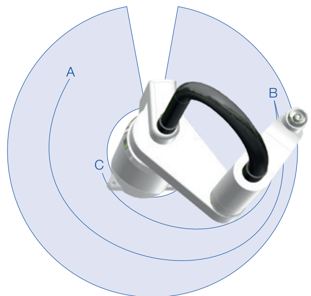
Herkömmliche SCARA-Roboter: Nierenförmiger Arbeitsbereich mit Totzone
